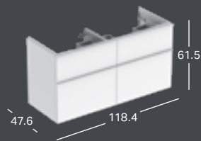
GEBERIT ICON UNDERSKÅP FÖR DUBBELTVÄTTSTÄLL, MED FYRA LÅDOR
